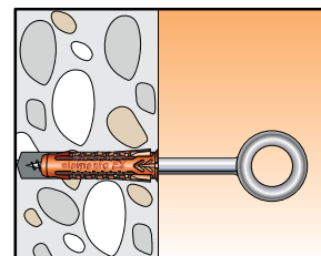
4. Крепление установлено
